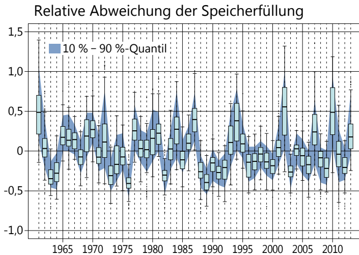
Pflanzenverfügbare Bodenwasserspeicherfüllung in der Vegetationsperiode für die BZE II-Punkte in Sachsen-Anhalt im Zeitraum 1961 bis 2013. Verteilung (Median, Quantil-Bereich (25-75 %, 10%- und 90 %-Quantil) dargestellt als relative Abweichung vom Mittelwert des Zeitraums 1961 bis 1990.
